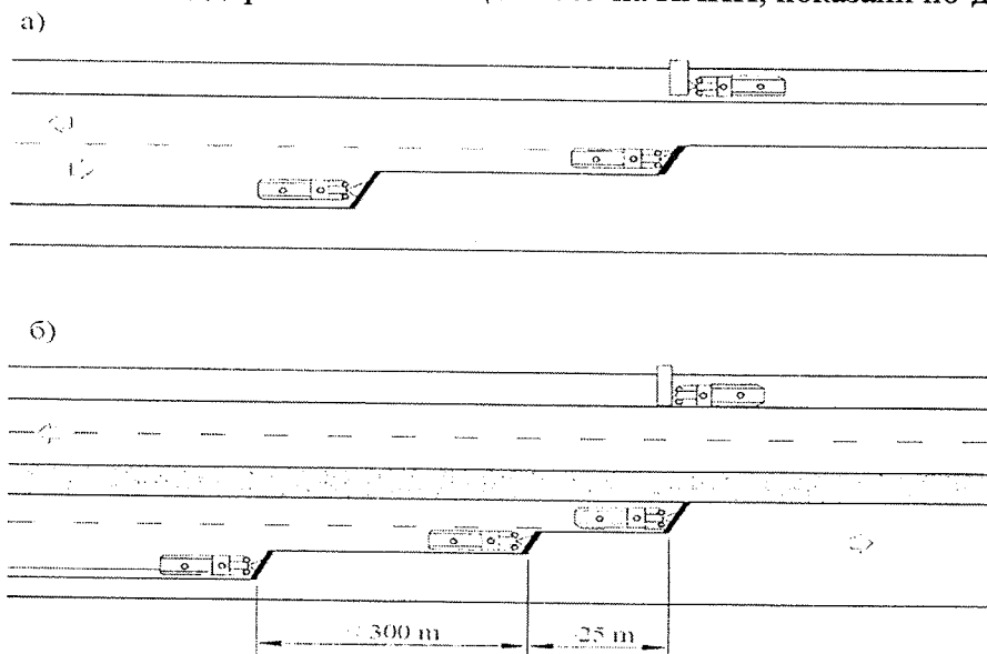
а) – при двупетовни пътища; б) – при автомагистрала
