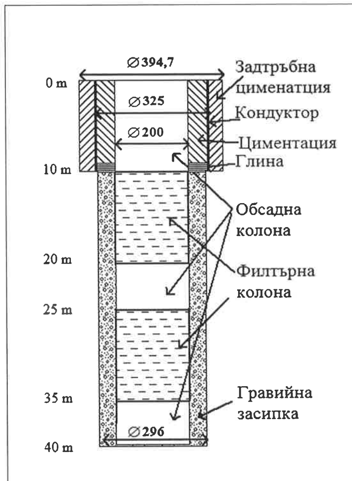
Фиг.1. Проектна конструкция на тръбен кладенец
